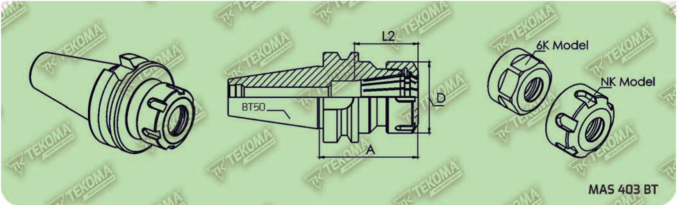
BT50 Pens Başlığı
